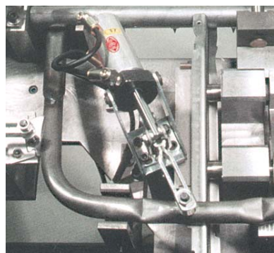
Dispositivo de solda - Grampo 810-UF
