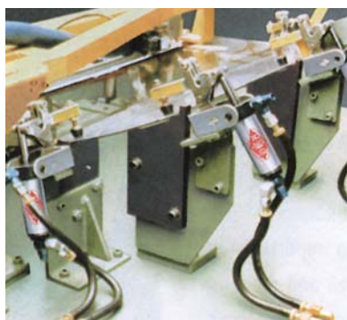
Dispositivo de fixação de placa de acrílico Grampo 817-UF
