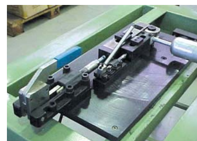
Dispositivo de montagem - Grampo 504
