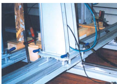
Equipamento de teste de durabilidade para móveis - Grampo 500
