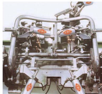
Dispositivo de montagem - Grampo 810-U
