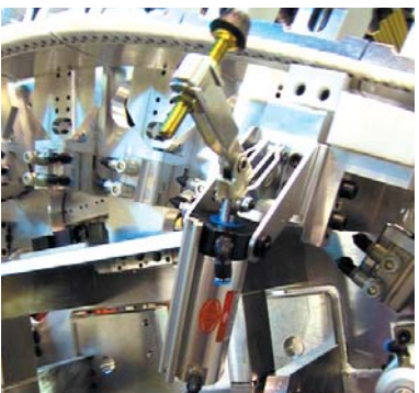
Dispositivo de montagem Grampo Pneumático 812-MR
