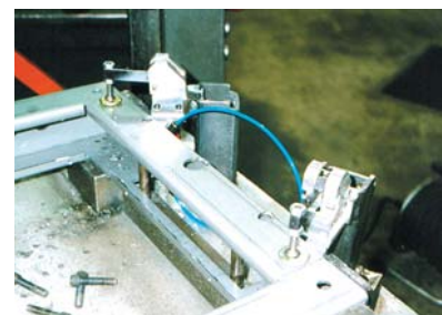
Dispositivo de montagem Grampo Pneumático LV8 113-DS
