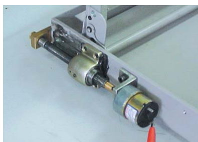
Movimentação de console de TV em ônibus e avião - Fusos rápidos modificados
