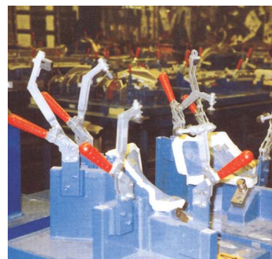
Dispositivo de solda - Grampo 210-U
