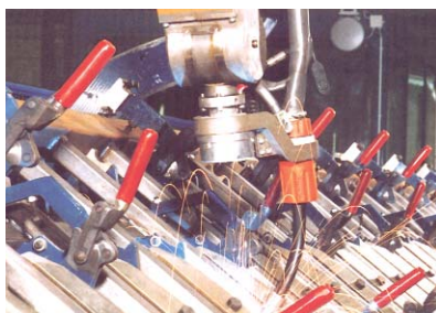
Dispositivo de solda robotizado Grampo CF-1165-I
