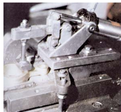
Dispositivo de usinagem - Grampo 807-UF
