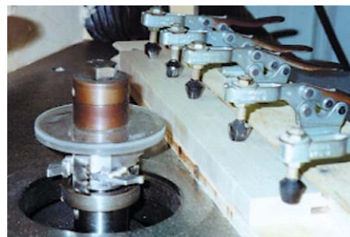
Usinagem de madeira com tupia Grampo 225-U
