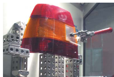
Sistema de medição - Grampo 210-U
